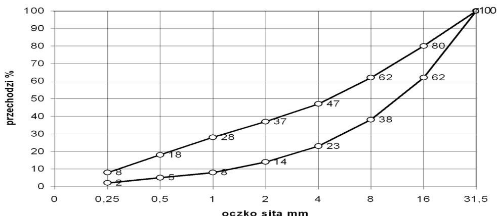
Rysunek 2. Graniczne krzywe uziarnienia kruszywa 0+31,6 mm (dla betonu klasy B25)
