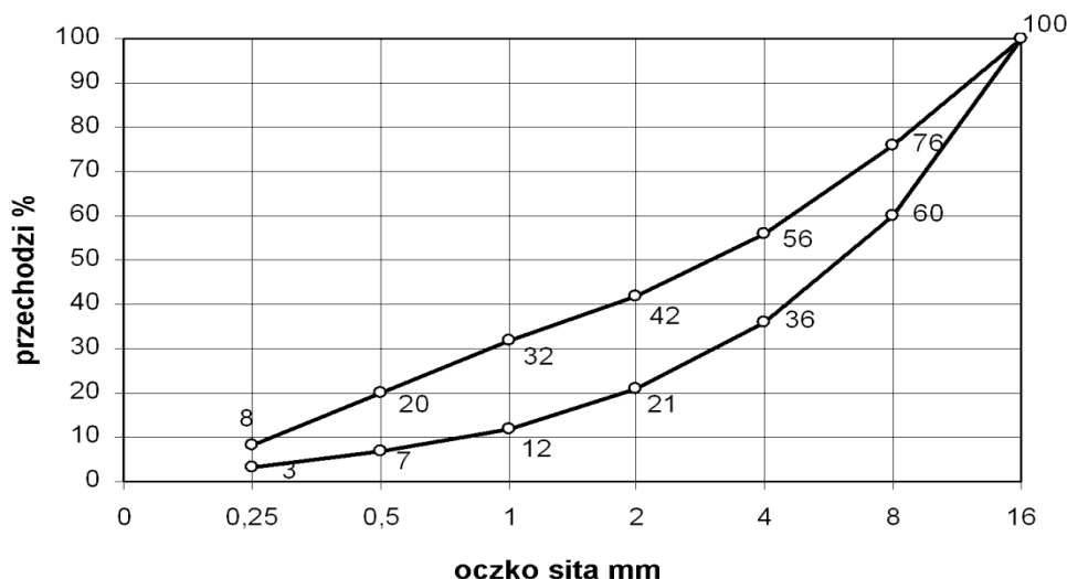
Rysunek 1. Graniczne krzywe uziarnienia kruszywa 0 ÷ 16 mm (dla betonu klasy B30)
