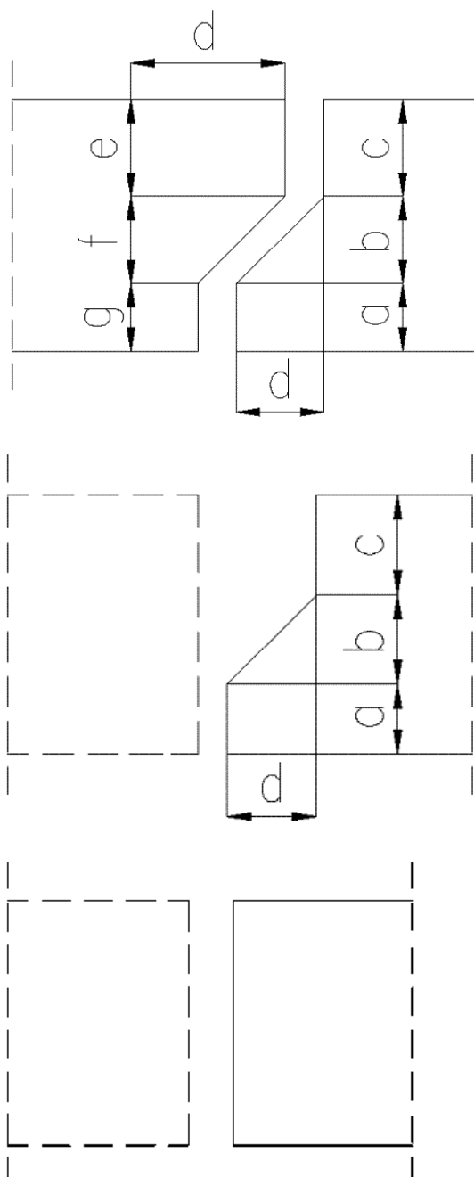
Rys.1. Typowe złącza między elementami prefabrykowanymi przepustów
