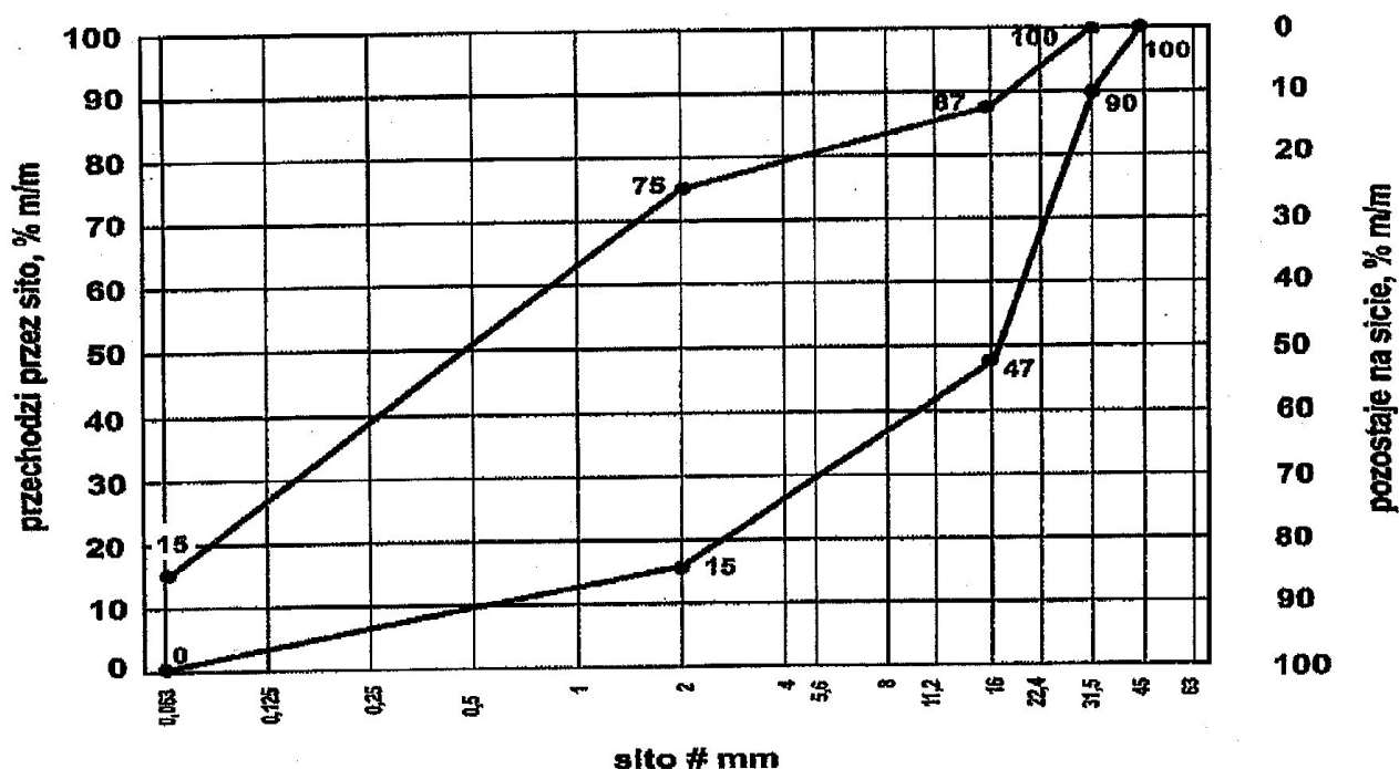
Rys. 2.6.3. Uziarnienie mieszanki niezwiązanej 0/31,5 do nawierzchni
