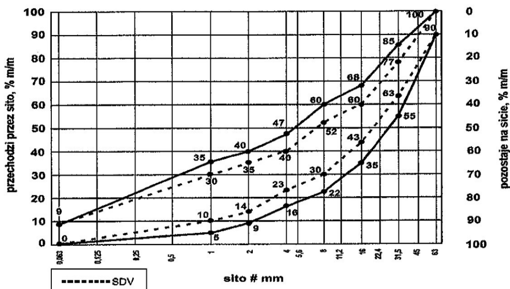
Rysunek 2c. Uziarnienie mieszanki niezwiązanej 0/63 do podbudowy zasadniczej
