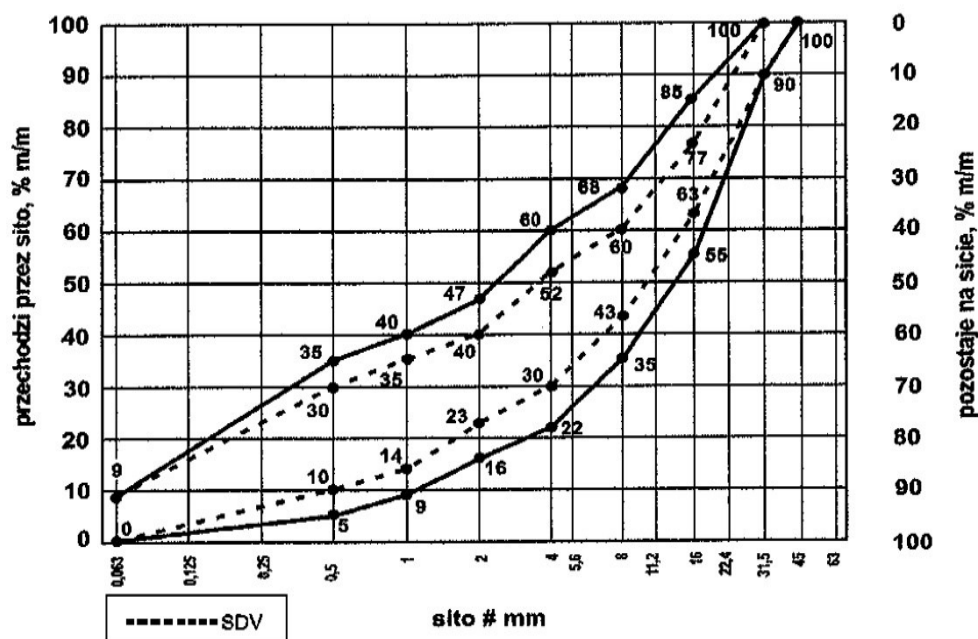
Rysunek 2a. Uziarnienie mieszanki niezwiązanej 0/31,5 do podbudowy zasadniczej
