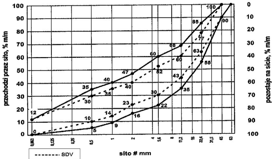
Rysunek 1c. Uziarnienie mieszanki niezwiązanej 0/63 do podbudowy pomocniczej
