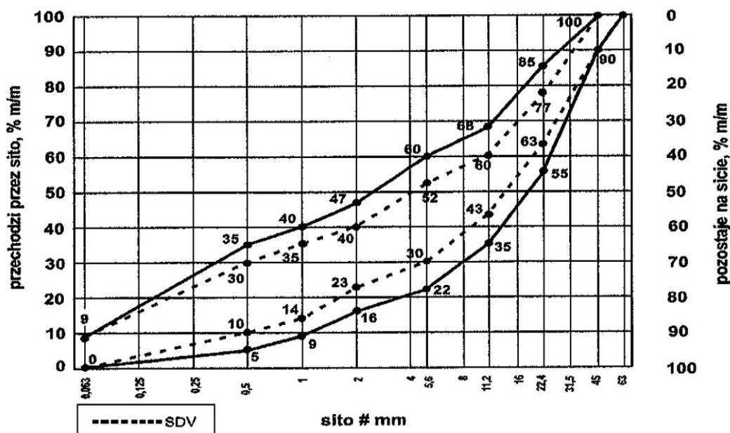
Rysunek 2c. Uziarnienie mieszanki niezwiązanej 0/63 do podbudowy zasadniczej
