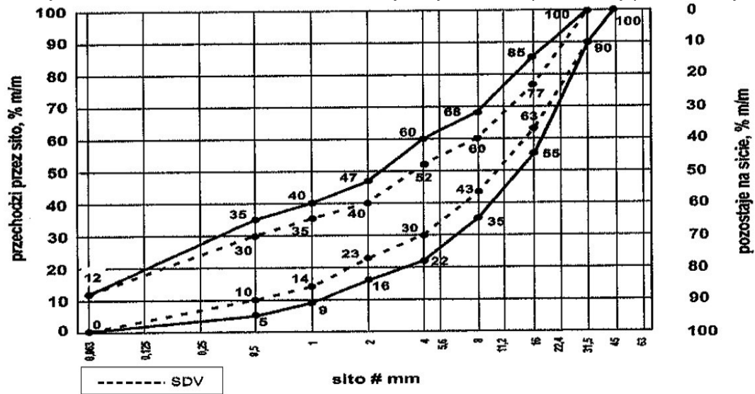
Rysunek 1b. Uziarnienie mieszanki niezwiązanej 0/45 do podbudowy pomocniczej
